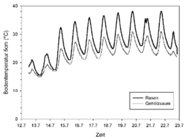
Bodentemperaturen in 5cm Tiefe, Juli 2007
